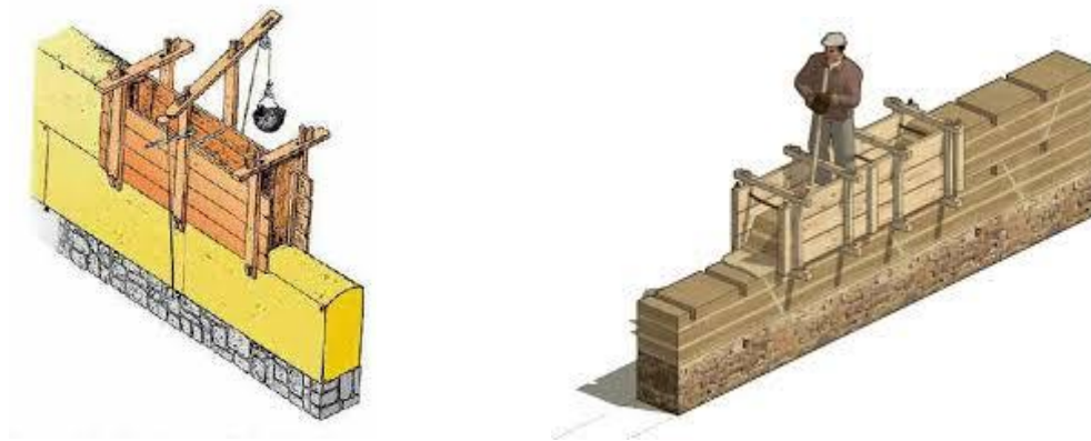
Formas sencillas de hacer paredones con barro prensado
